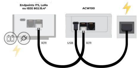
Alimentação via fonte externa USB
