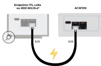
Alimentação via cabo RJ11
